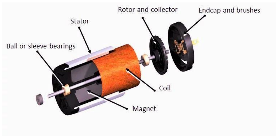
Image 2 : Composants d'un moteur CC sans fer
